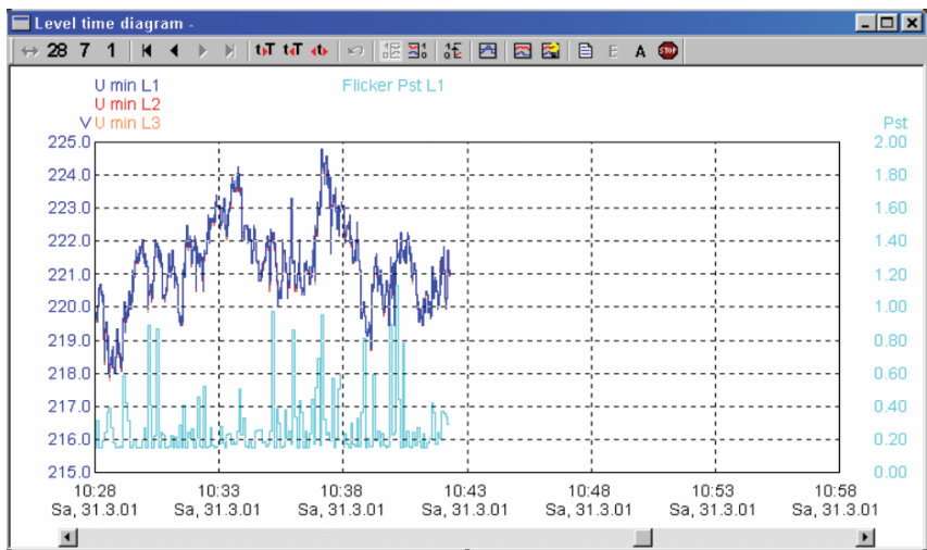
图 15. 实时读数 (联机测试)
