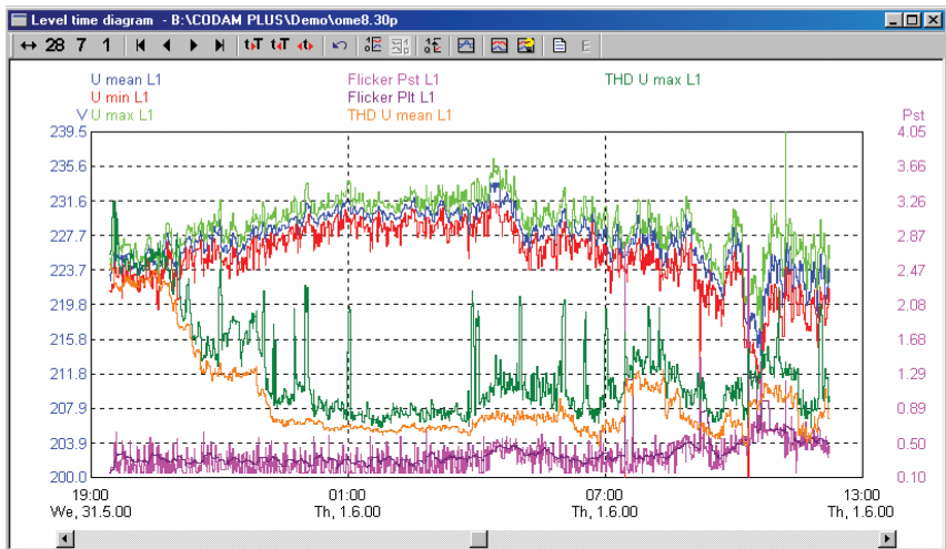
图 17. 时间曲线示意图
