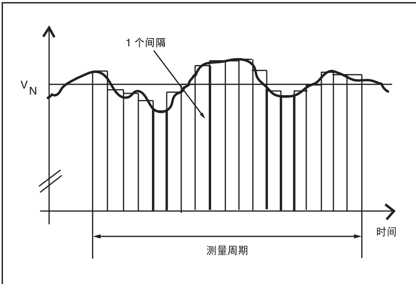
图 10. 测量电压变化
