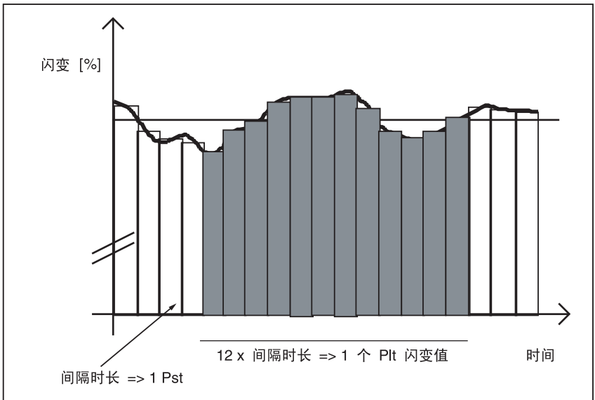
图 14. 测量闪变值
