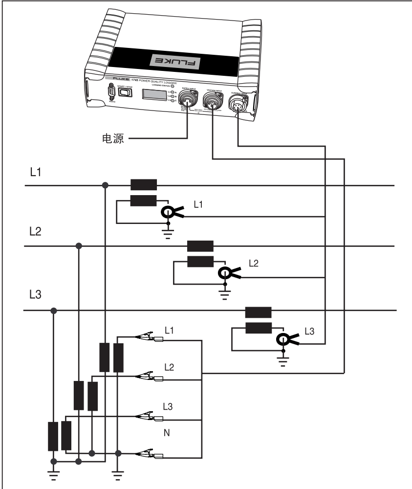
图 7. 在三线制（三角形）系统中用三个电压转换器测量三相电压
