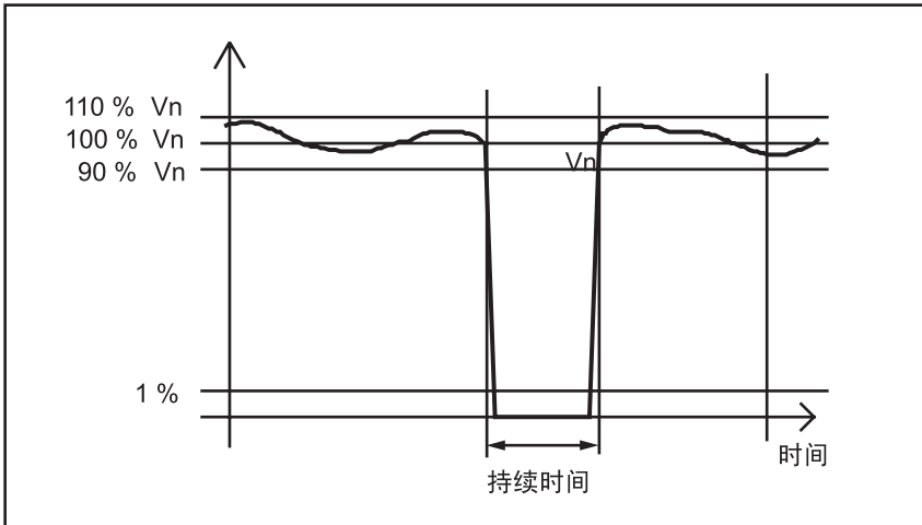
图 12. 电压中断
