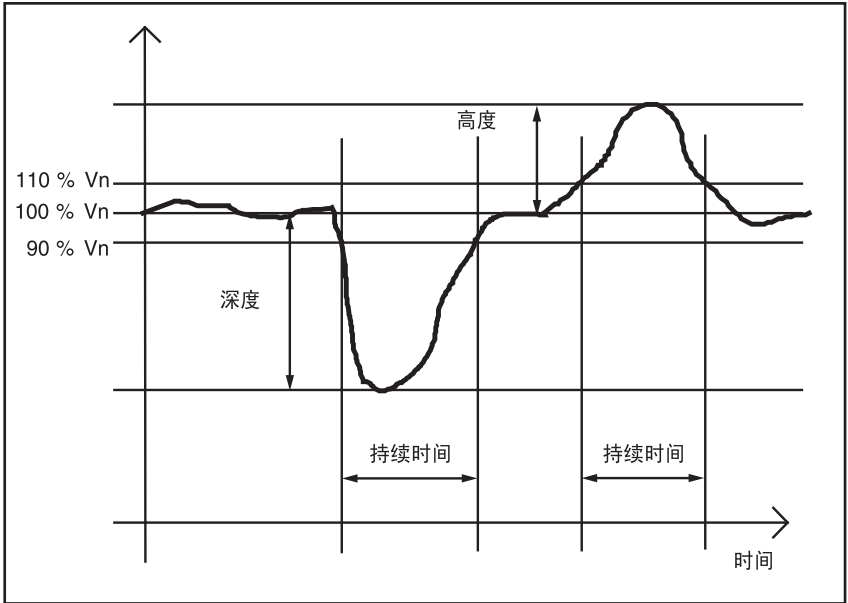
图 13. 电压骤降与骤升
