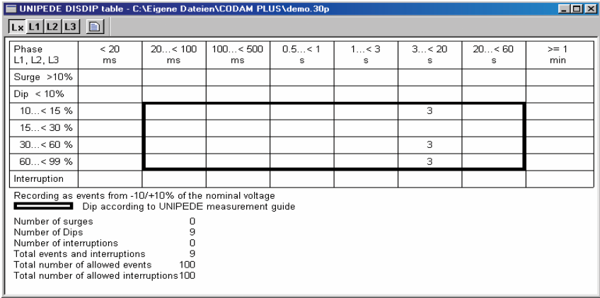
图 18. UNPEDE DISDIP 表
