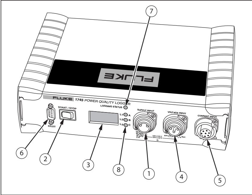
图 2. 1745 型电力质量记录仪 — 正视图
