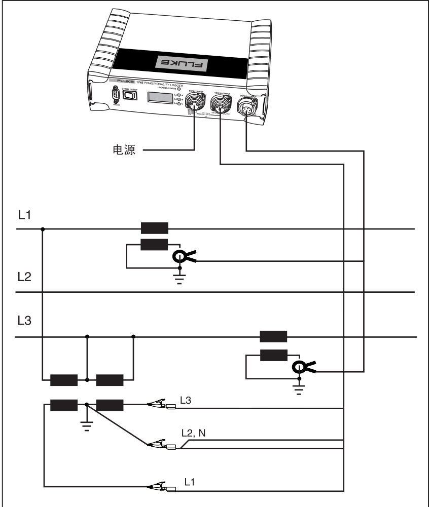
图 8. 二元三角形连接
