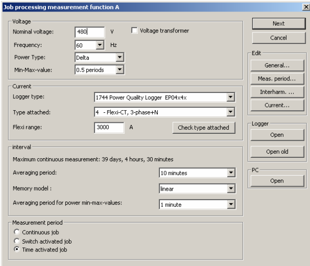
图 9. 记录仪的基本设置参数
