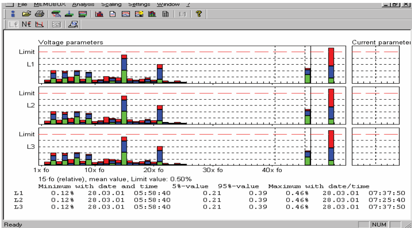
图 19. 电压和电流谐波的累积频率
