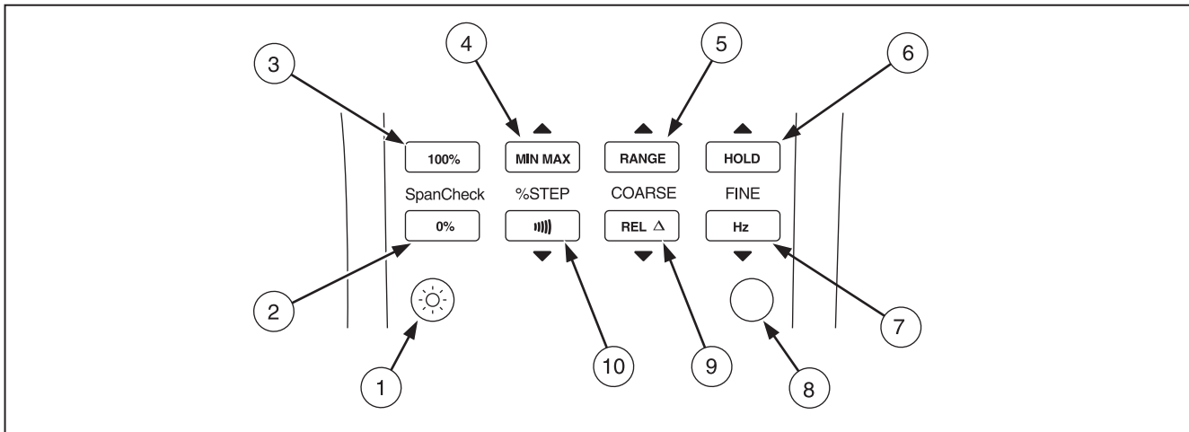
图 5.按键
