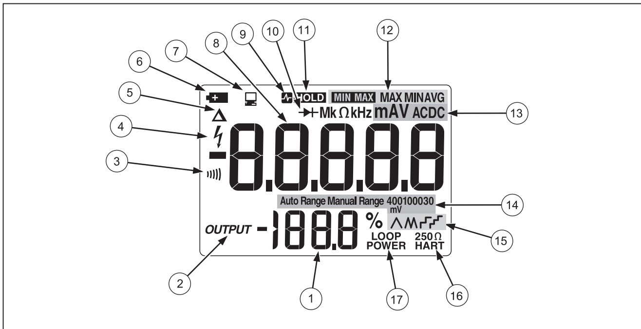
图 6.显示单元
