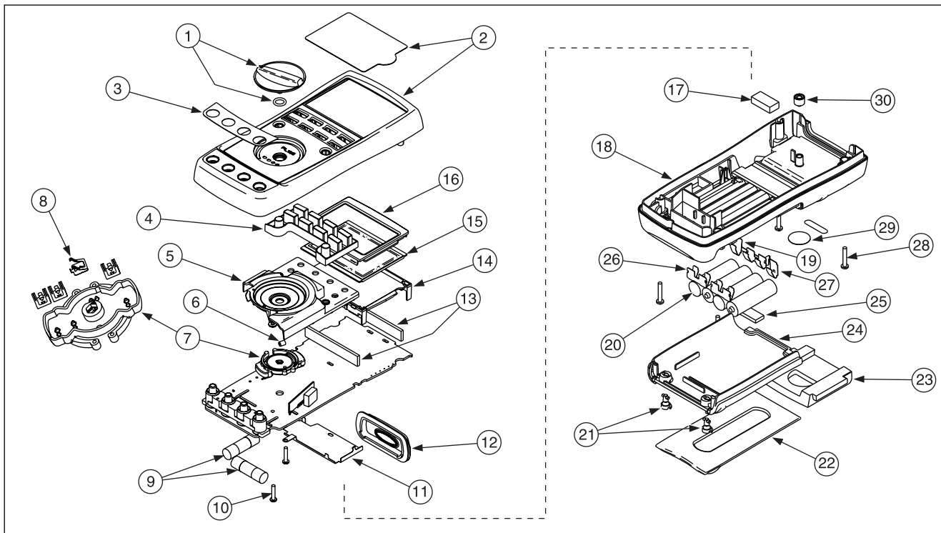
图 12.更换零件
