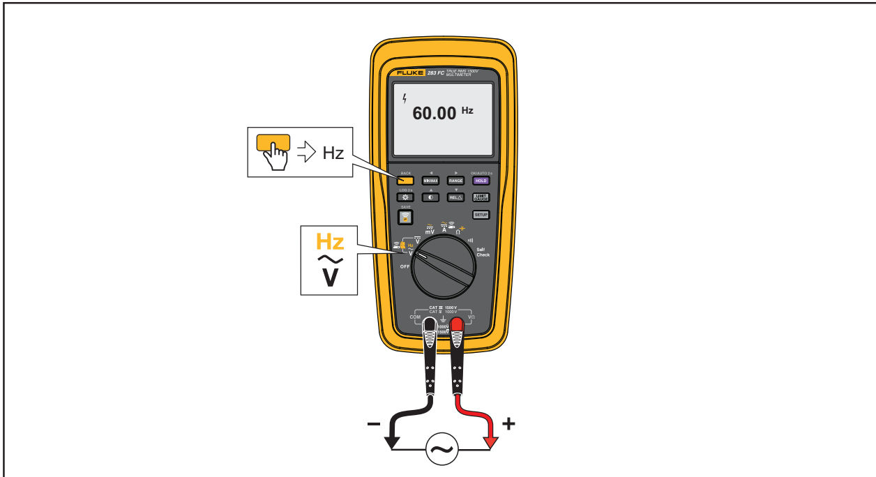
图 6. 频率测量
