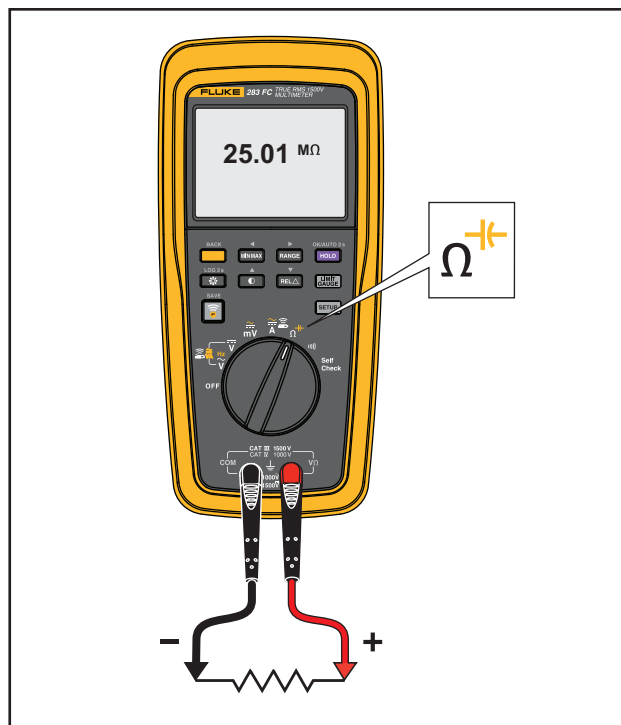
图 3. 电阻测量
