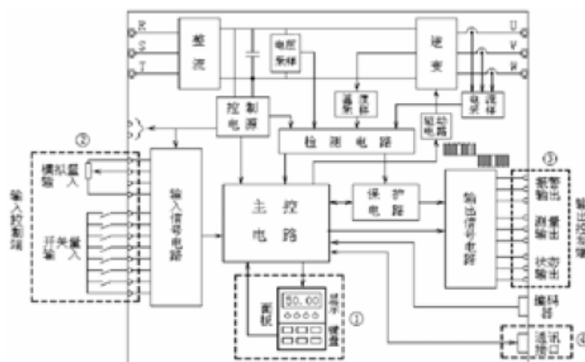
圖 1. 典型的伺服控制電路
