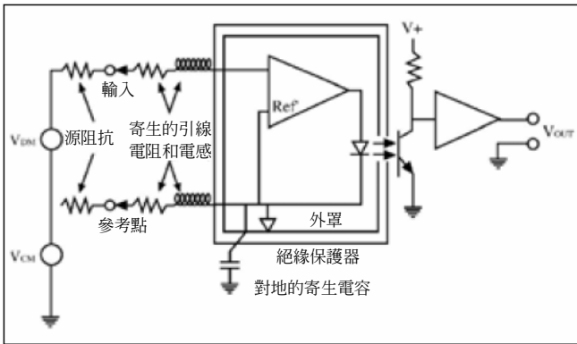
圖 11. 隔離外殼產生的不平衡輸入電容。由此形成的交流分壓器使得探棒夾子處的 V_{ref} \neq V_{ref}
