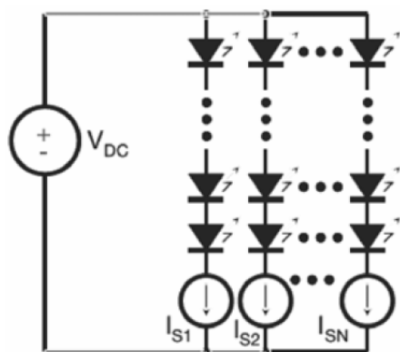
圖 17. LED 恆流源背光驅動器
