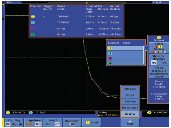
圖 8. 手動消除電壓探棒與電流探棒間的時脈偏移
