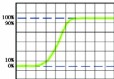
■ 1X 被動式探棒的上升時間波形
