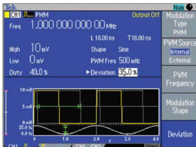
圖 6. AFG3000 的 PWM 訊號輸出功能
