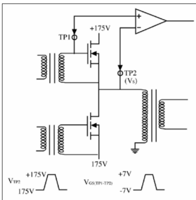
圖 7. 用來量測逆變器橋電路上上部電晶體的開極 - 源極電壓的差動放大器。注意在量測過程中，源極電位變化了 350V。
