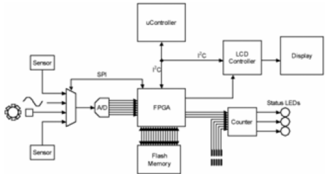
圖 8. 控制系統方塊圖
