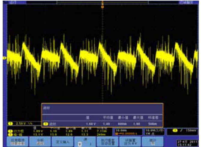
圖 4. 儲能電容的漣波量測
