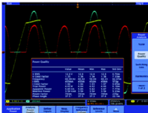
具DPO4PWR的Tektronix MSO/DPO4000示波器
