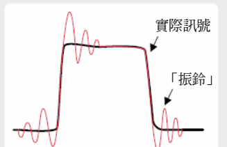
▶ 寄生電感和電容導致的振鈴使訊號失真，使量測無效
