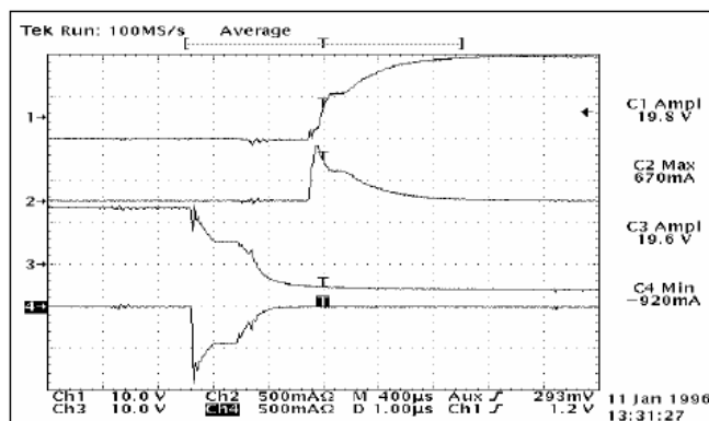
量測 IGBT 電流和電壓波形
