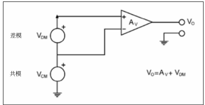
圖 6. 差動放大器
