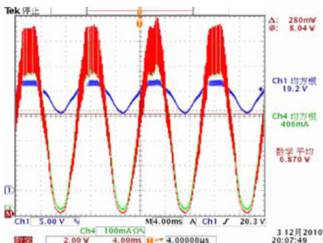
圖 5. 示波器使用暫態功率積分法量測輸出功率
