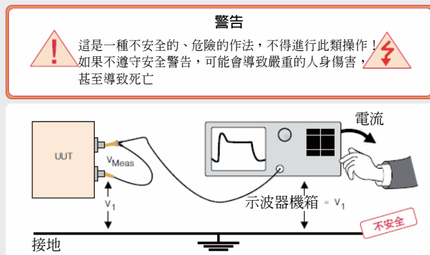
▶ 浮動量測，危險電壓發生在示波器機箱上。V1 可能有幾百伏！
