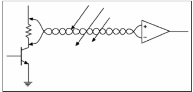
圖 16. 將輸入引線絞扭在一起，迴路面積非常小，故穿過其中的磁場較少。感應電壓往往出現在 VCM 通道，可以被差動放大器抑制。
