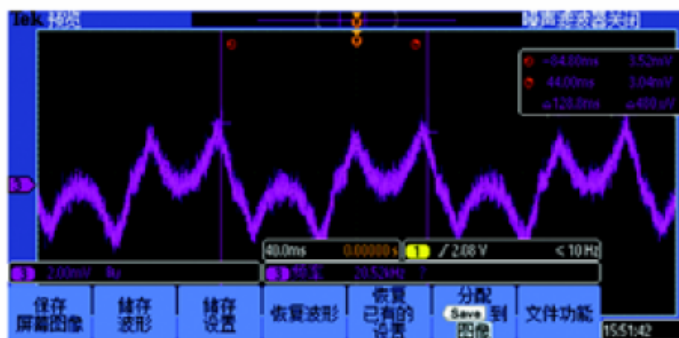
SVPWM 調變控制下輕載狀態的電流波形
