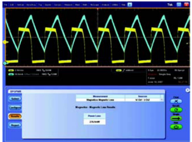
圖 16. 使用 DPOPWR 所測得之單線圈電感的功率耗損
