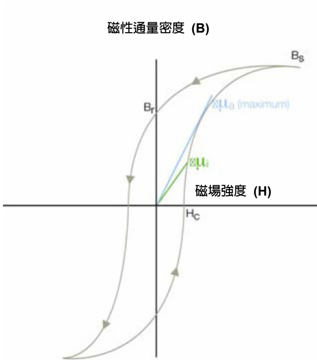
圖 17. 磁性元件的一般 B-H (磁滯) 圖
