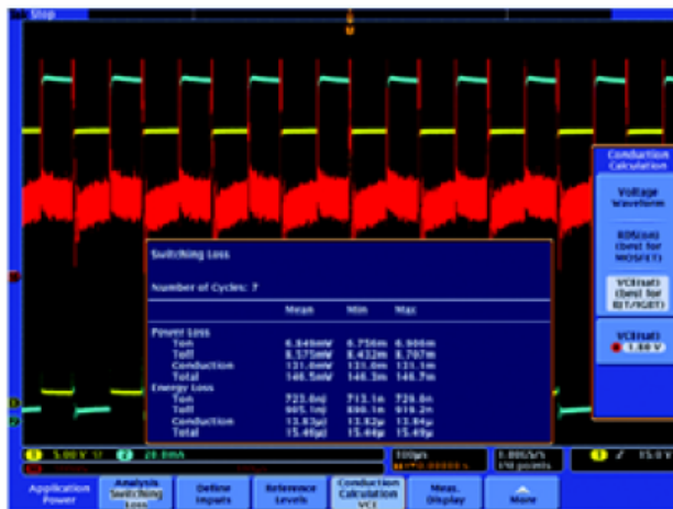
具 DPO4PWR 模組的 Tektronix MSO/DPO4000 示波器
