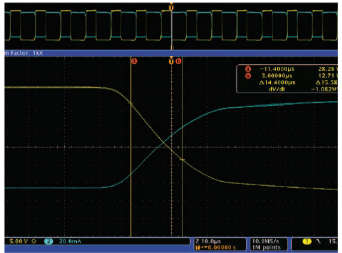
圖 15. DPOxPWR 迴轉率量測
