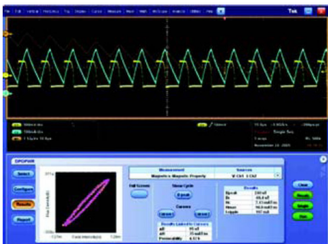
圖 19. 單線圈電感的 B-H 圖
