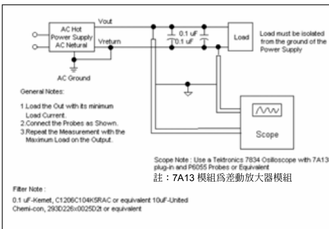
圖 2. INTEL 建議的 PARD 差動檢測連接圖
