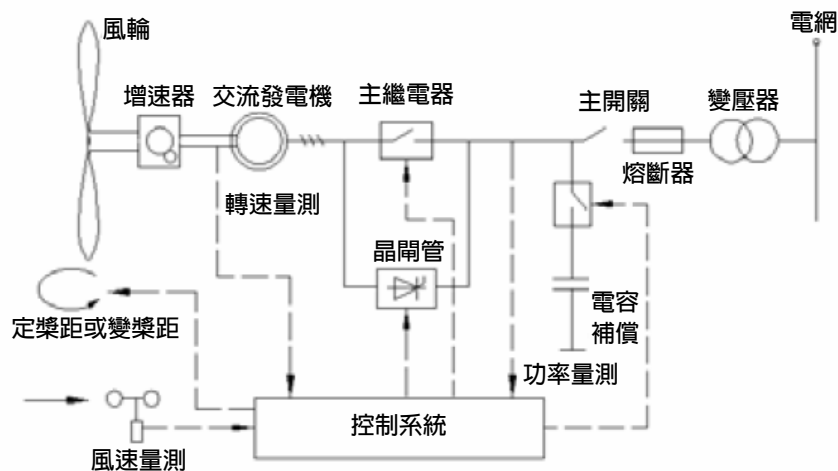
並網運行的水平軸風力發電機組的原理方塊圖
