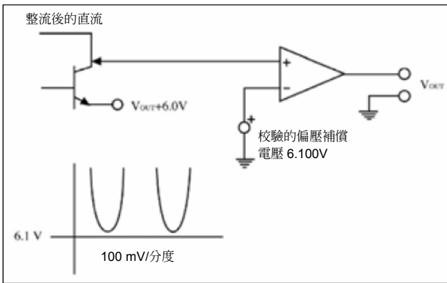
圖 12. 用校驗的偏壓補償準確量測輸出穩壓器集電極上的電源漣波谷。注意：示波器設定在 100mV/分度，地電位在螢幕外 61 個分度。
