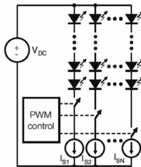
圖 19. 具有調變電流源的背光 LED 驅動器
