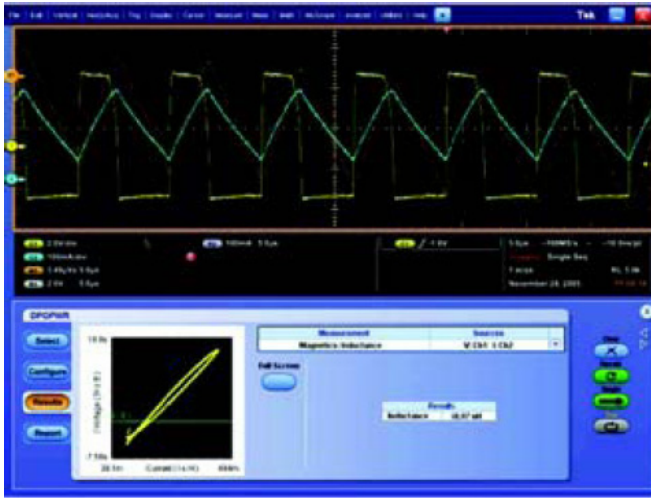
圖 14. DPOWPR 應用軟體所產生的電感量測
