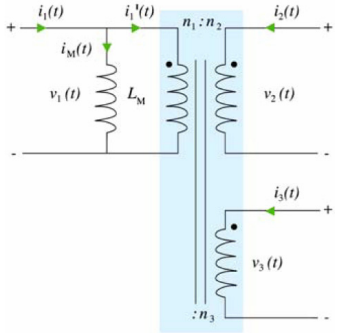
理想的變壓器
