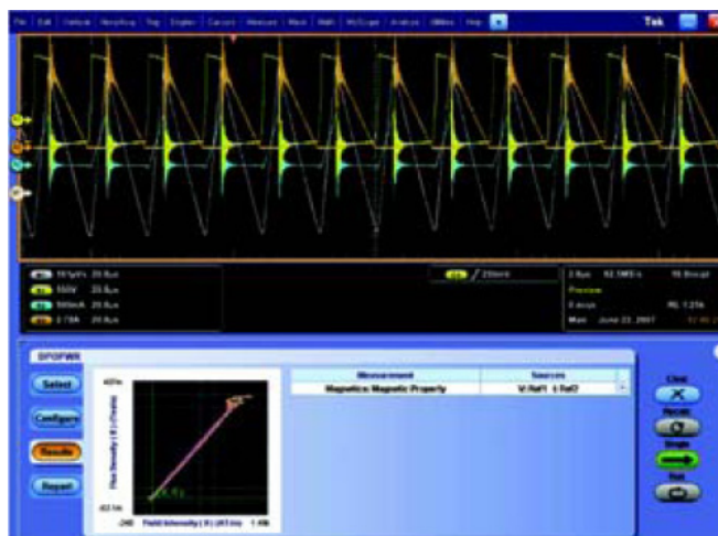
圖 20. 變壓器的 B-H 圖
