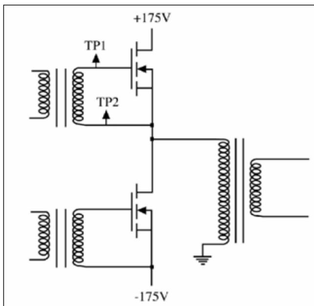
圖 1. 在測試點 TP1 和 TP2 之間量測交換式電源供應器中的閘極驅動訊號。兩點都沒有接地。
