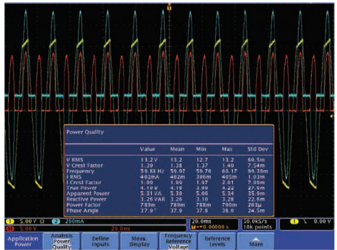
圖 12. DPOxPWR 電源品質量測
