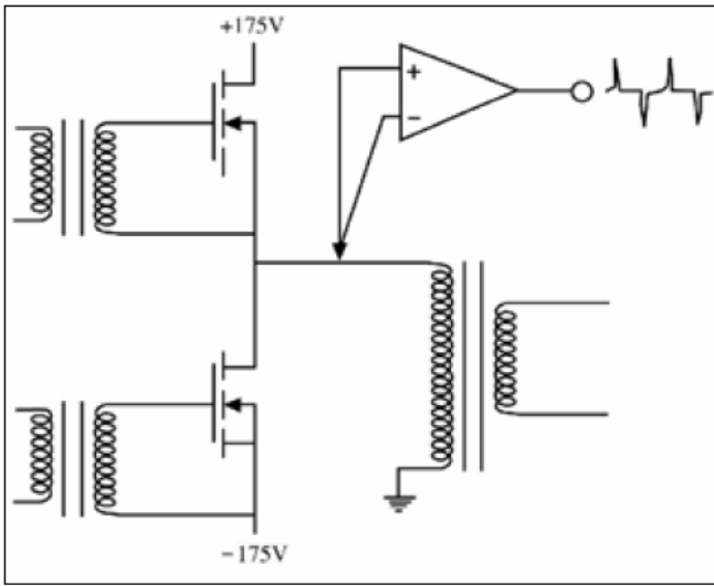
圖 9. 對共模抑制進行試驗測試。由同一點驅動兩個輸入端。殘留的共模出現在輸出端。此項測試沒有發現不同的源極阻抗的影響。
