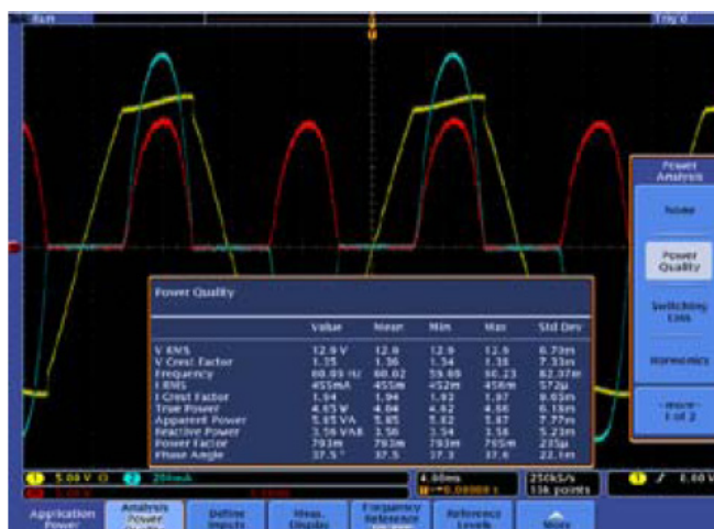
圖 1. 電源品質參數測試
