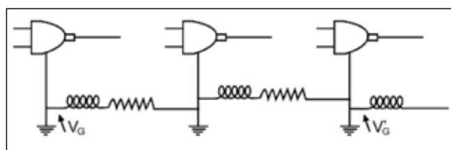
圖 5. 接地佈線系統中的微小寄生電感和電阻導致 V_G \neq V'_G
