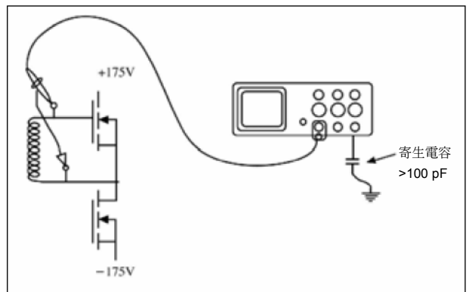
圖 10. 即便示波器處於「浮動」狀態，寄生電容也會形成交流分壓器，從而增加量測的誤差。注意：反轉的探棒引線會爲閘極增加 >100 pF 的電容，有可能破壞電路。
