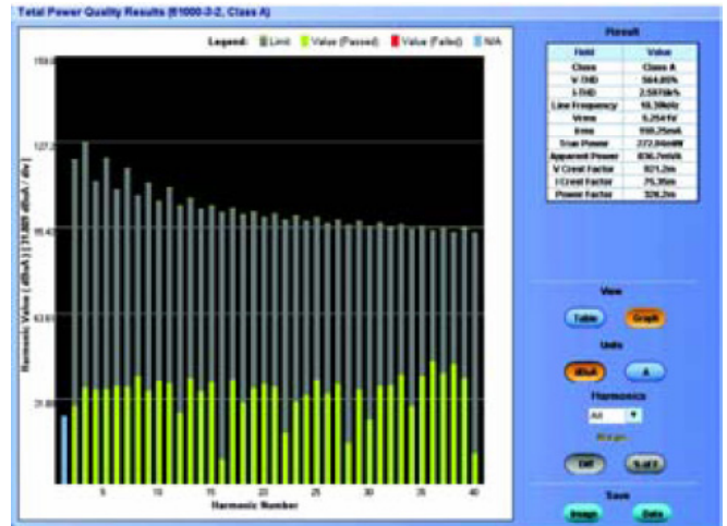
圖 22. 使用 DPOPWR 量測和分析軟體獲得的電源品質結果, 量測規格包括真實功率、視在功率、波峰因素、總諧波失真、功率因素及電流諧波直方圖。
