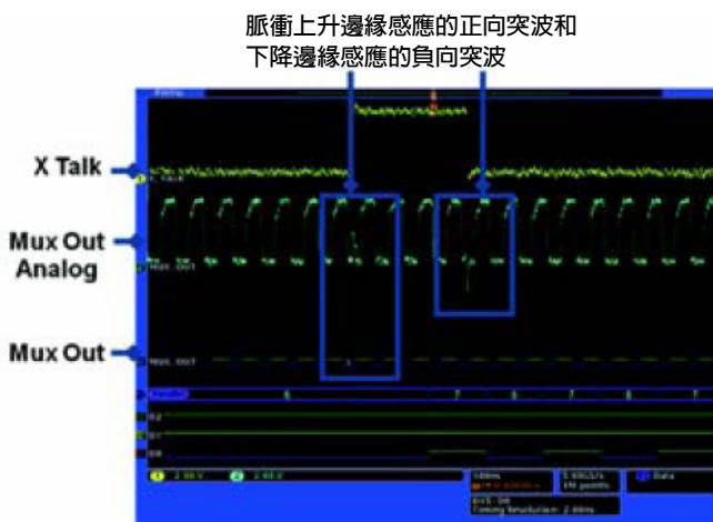
圖 11. 發現串音
