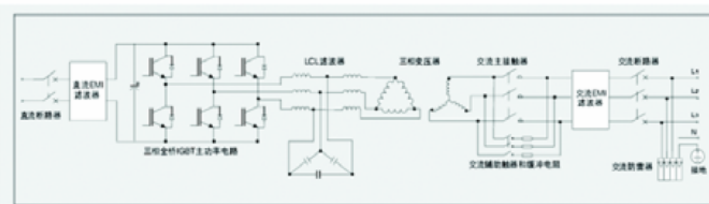
採用功率頻率變壓器隔離的大功率三相並網逆變器
