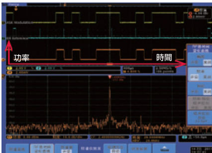
功率隨時間變化顯示
