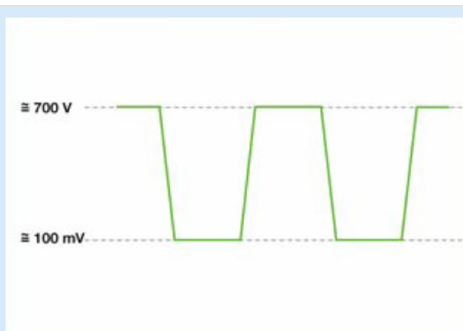
圖 6. 切換裝置上的一般訊號
