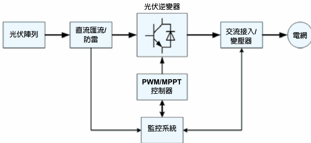
並網型 (主動式逆變) 光伏電站構成原理圖
