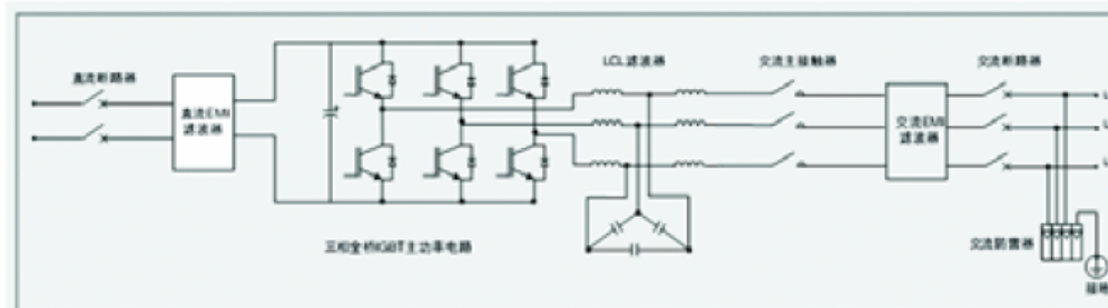
無變壓器隔離的大功率三相並網逆變器 (輸出電壓可以從 270 V~400 V)
