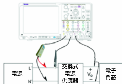
電壓驟降
