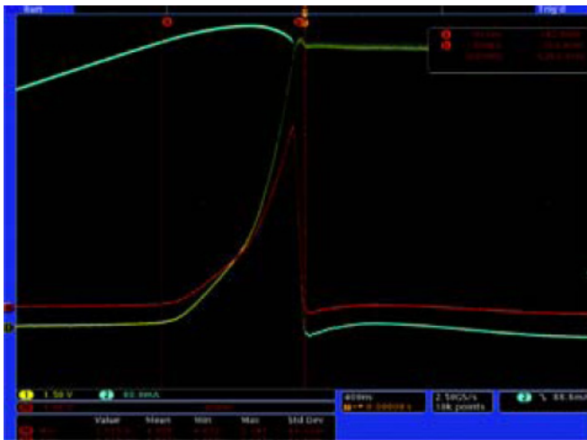
圖 10. 在這一偏移下，功率波形的峰值振幅是 4.958 W
