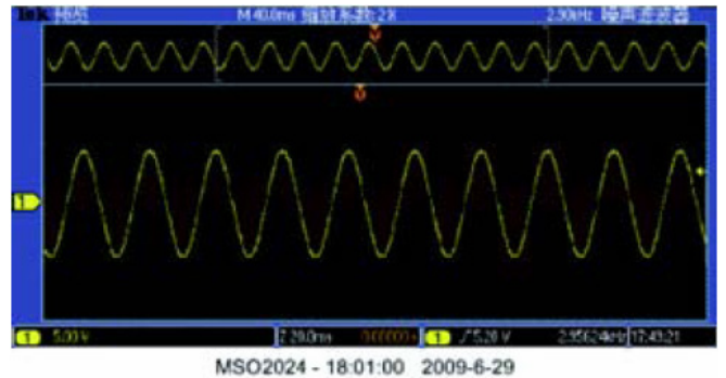
圖 5. 驅動輸出電壓訊號 SPWM 基波測試
