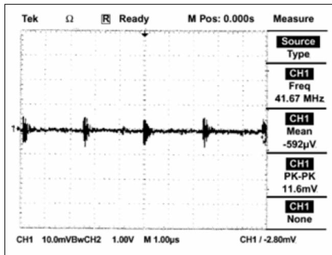
圖 1. 交換式電源供應器的輸出雜訊波形
