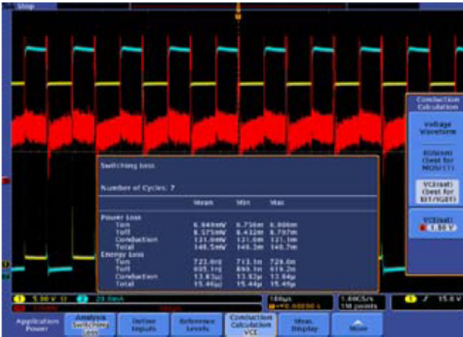
圖 2. MOSFET 切換損耗測試
