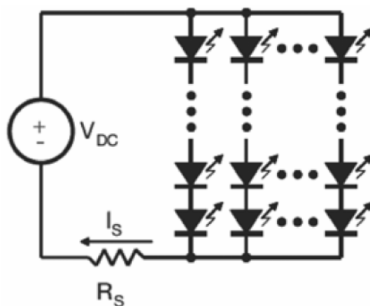
圖 18. LED 背光驅動器，配備限流電阻
