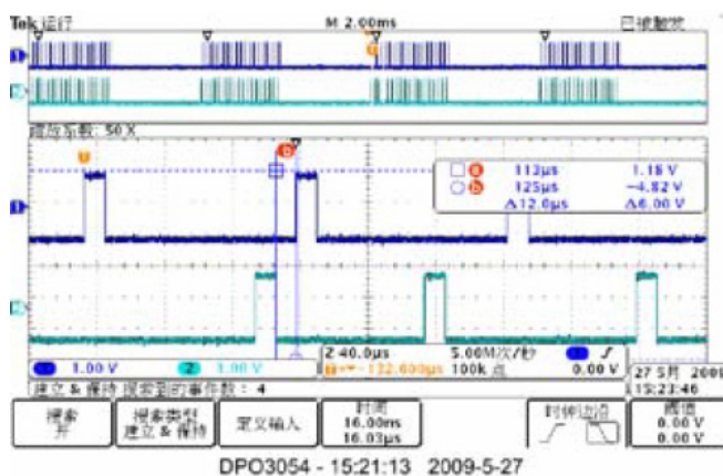
圖 2. 波形搜尋功能自動找到死區時間不足的同橋臂驅動脈衝組
