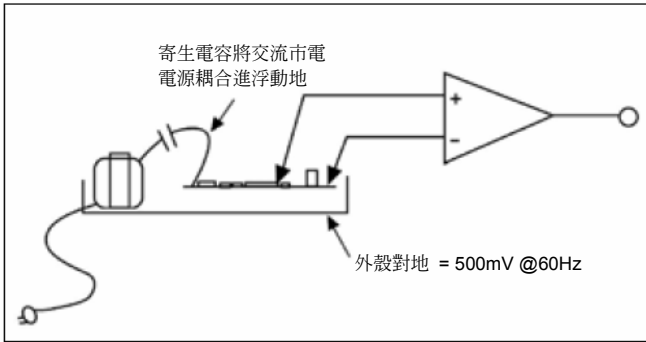
圖 18. 消費性音訊電子元件中的 VCM。這些設備通常使用雙芯電源線，其機箱和電路都是浮動的。
