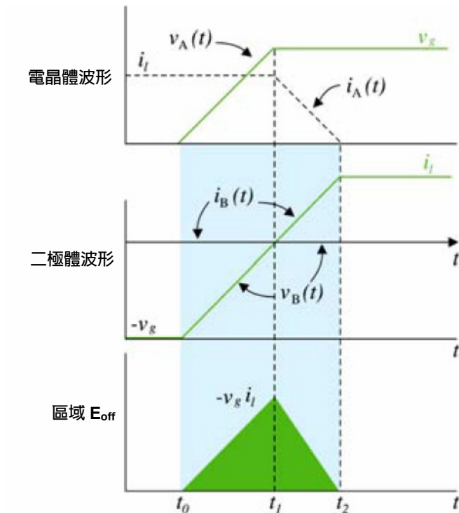
圖 2. 計算關閉耗損
