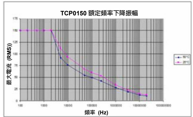
圖 3. 施加大於最大連續電流的電流時間不要超過 10 秒，以將加熱效應降到最小。
