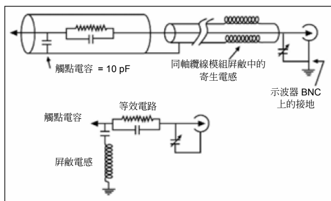
圖 3. 探棒觸點電容和接地電感形成的串聯諧振電路。
