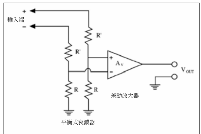
圖 14. 具衰減器的差動放大器簡圖
