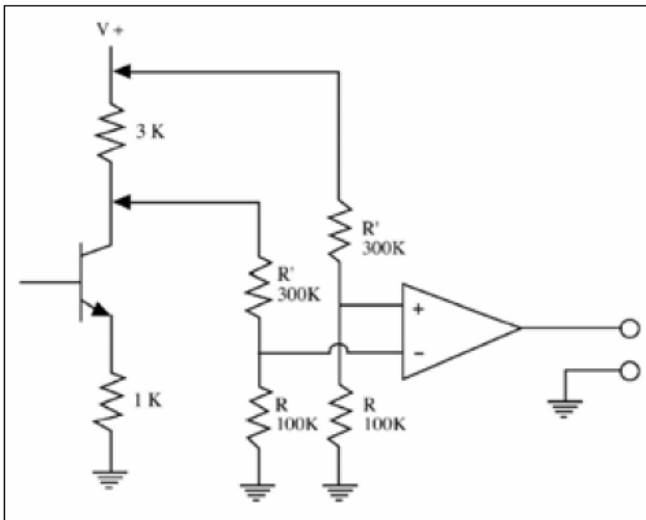
圖 17. 源阻抗不平衡所造成的影響。+ 輸入衰減器是從 0\ \Omega 驅動的，但輸入衰減器是從 3\ \text{k}\Omega 以下驅動的。結果與 900\ \text{k}\Omega 相加，使衰減增加而 CMRR 降低。
