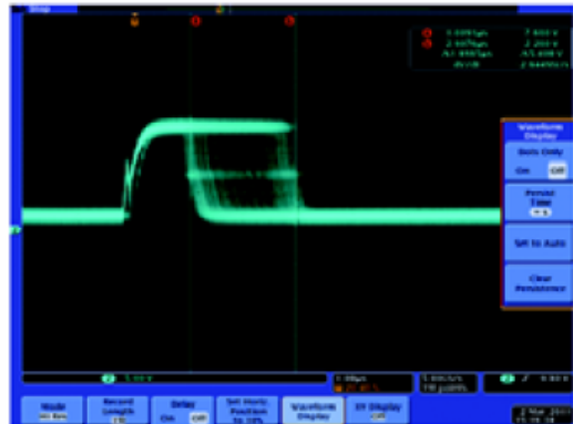
以持續累積功能觀察 PWM 訊號
