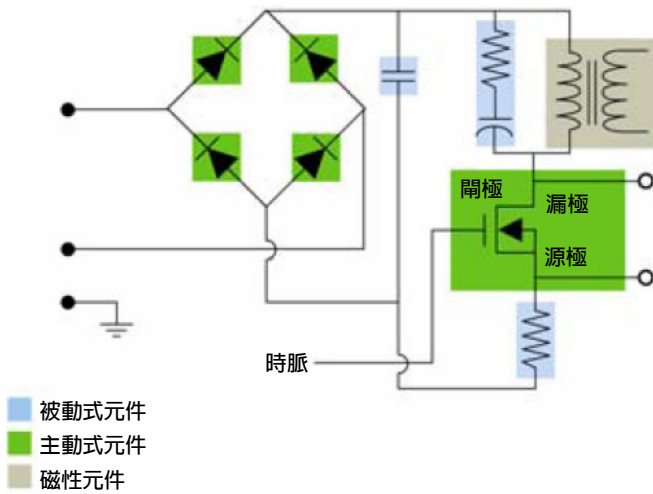
圖 1. 簡化的開關模式電源供應器線路圖
