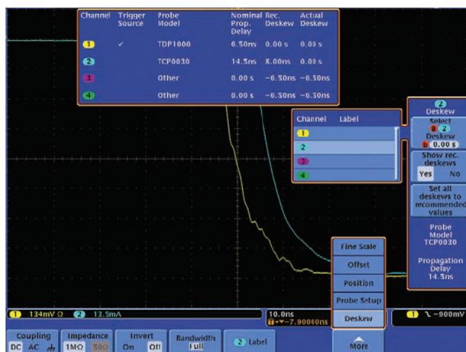
圖 5. 電壓與電流探棒間的預設時脈偏移
