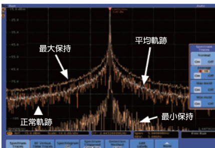
顯示 RF 訊號頻譜的四種常用軌跡
