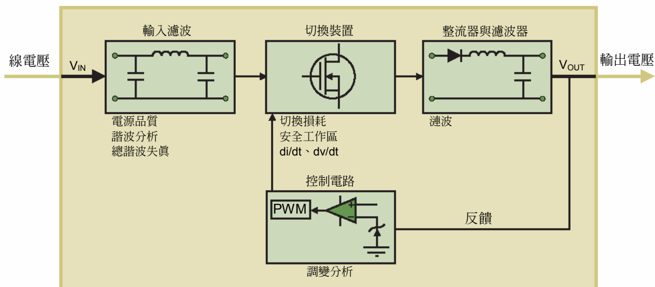
圖 1. 使用 DPOxPWR 功率分析軟體進行特性分析的 SMPS 元件
