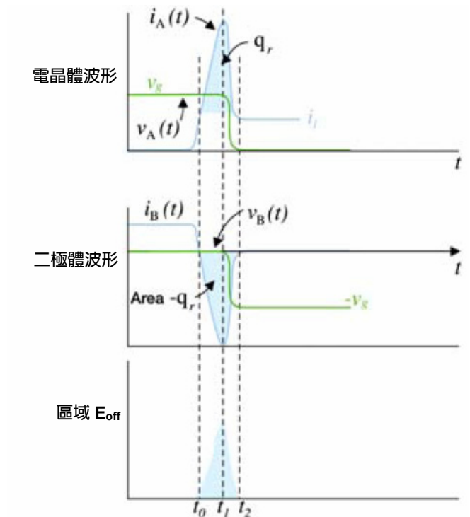
圖 3. 內含電容負載之 MOSFET 中的開啓耗損 2
