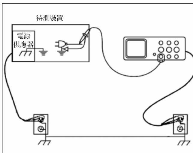
圖 2. 示波器探棒形成的接地迴路。示波器的金屬機箱和待測裝置連接到安全地線和內部公用電源線上。示波器探棒接地則透過輸入端 BNC 連接器連接到示波器機箱上。
