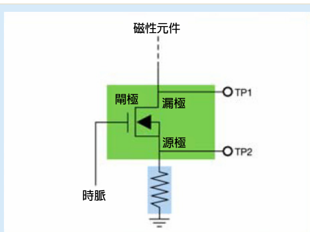
圖 5. MOSFET 切換裝置，顯示量測點
