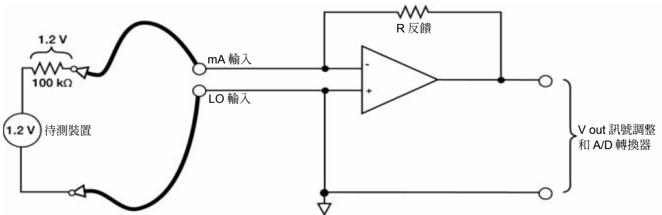
圖 2. 反饋 DMM 中的電路作為低電流安培計使用。Tektronix DMM4020 萬用電錶就是這樣一種工具。
