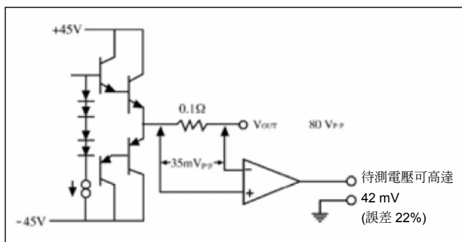
圖 8. CMRR 為 10,000:1 的差動放大器的共模誤差
