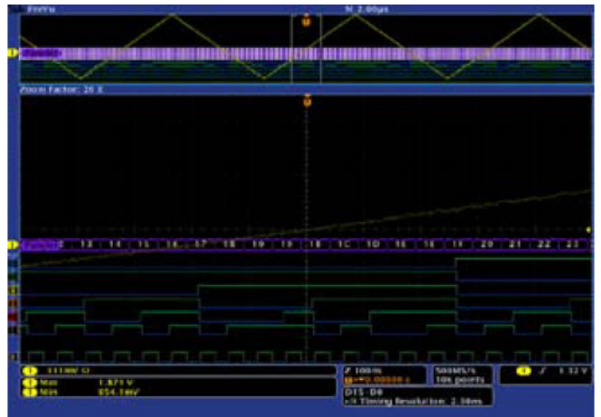
圖 5. 黃色感測器的類比訊號和 A/D 變換後的 6 位數位訊號以及轉換後的 16 進位資料
