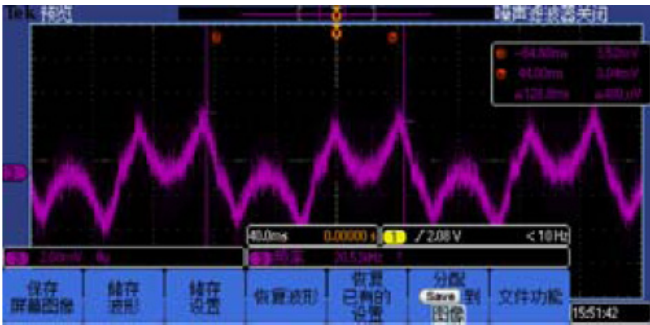
圖 3. SVPWM 調變控制下的輕載狀態電流波形
