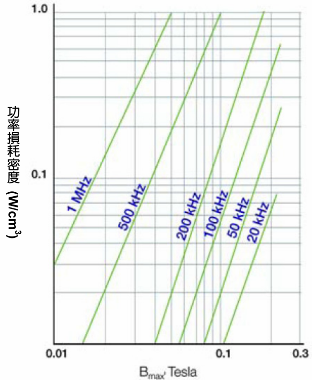
圖 15. 不同切換頻率下磁芯耗損對磁通量密度的分布圖
