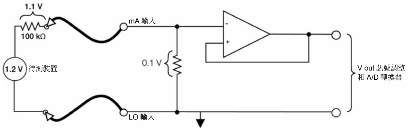
圖 1. 分流萬用電錶電路作為安培計使用
