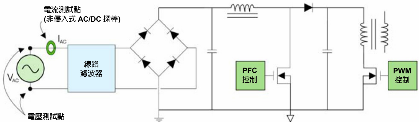
圖 21. SMPS 電源供應器 (只有主要部分) 及其電源品質測量測試點的簡圖。量測電源品質時，必須有同步輸入的 V_{AC} 和 I_{AC} 讀數。
