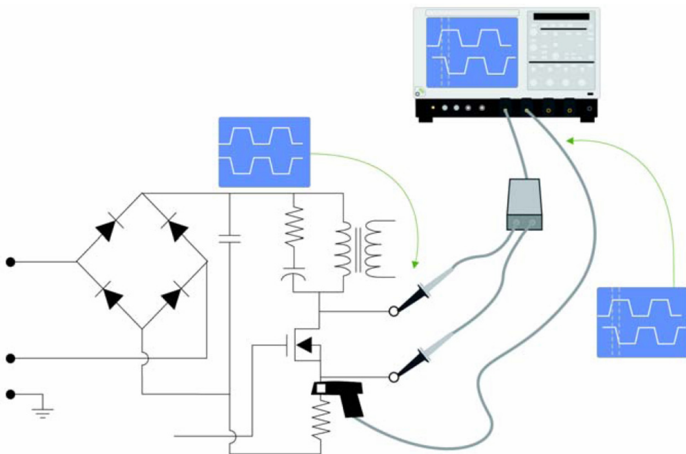
圖 8. 傳播延遲對電源量測的影響
