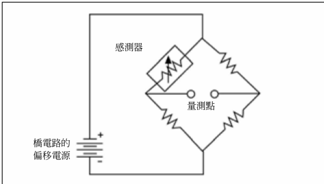
圖 13. 平衡橋電路中的感測器。在兩個分壓支路的抽頭之間進行差動量測。
