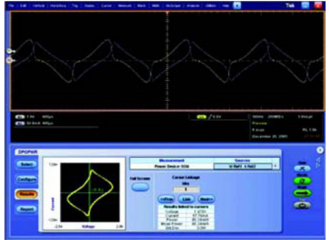
圖 4. 這個範例來自 DPO4104，說明 SMPS 的 SOA 標示圖。該標示圖可與切換裝置製造商所公佈的資料做比較。
