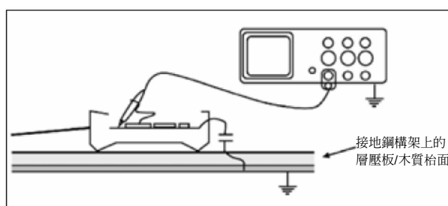
圖 4. 使用接地的示波器探測「浮動的」電池供電手機。手機電路和鋼製工作檯構架之間的電容對高頻率構成了虛擬接地迴路。
