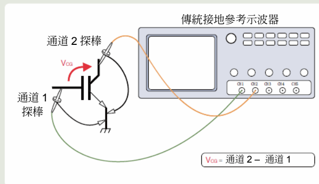
▶ 量測接地參考電壓的兩支探棒實例
