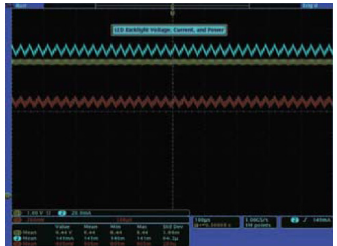
圖 21. 使用 MSO4000 系列示波器進行 LED 背光功率測試的顯示介面
