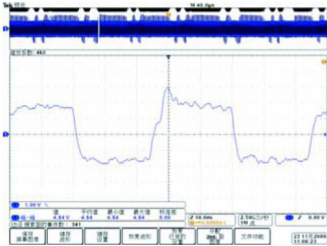
圖 6. 馬達驅動系統驅動電壓的過電壓突波擷取與分析
