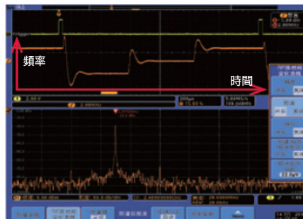
頻率隨時間變化顯示
