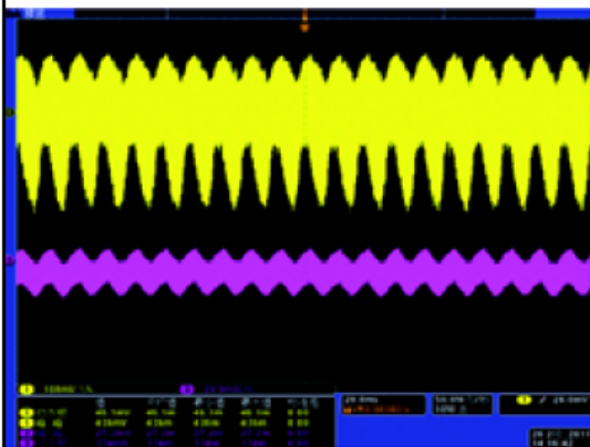
CH1：電壓漣波 CH3：電流漣波
