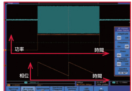
相位隨時間變化顯示
