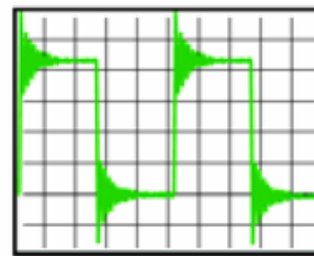
未接接地線
