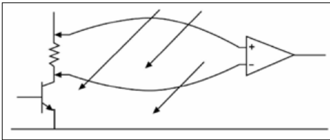
圖 15. 隨時間變化的磁場穿過間隔開的引線時感應出電壓，猶如變壓器的線圈。此電壓作為差動成分輸入放大器，並累加到真正的 VDM 訊號上。
