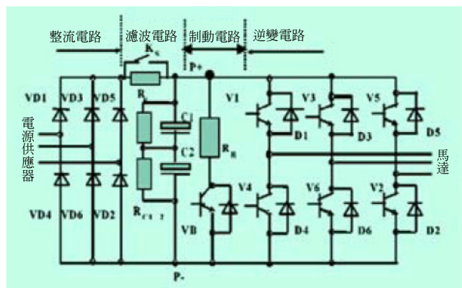
圖 1. 變頻器驅動電路方塊圖
