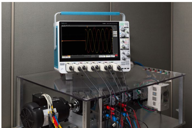
三相馬達啟動後會進行電壓量測，顯示三相輸入電壓。
