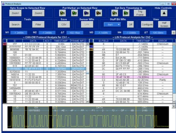
CAN 和 LIN 定时和协议解码。
